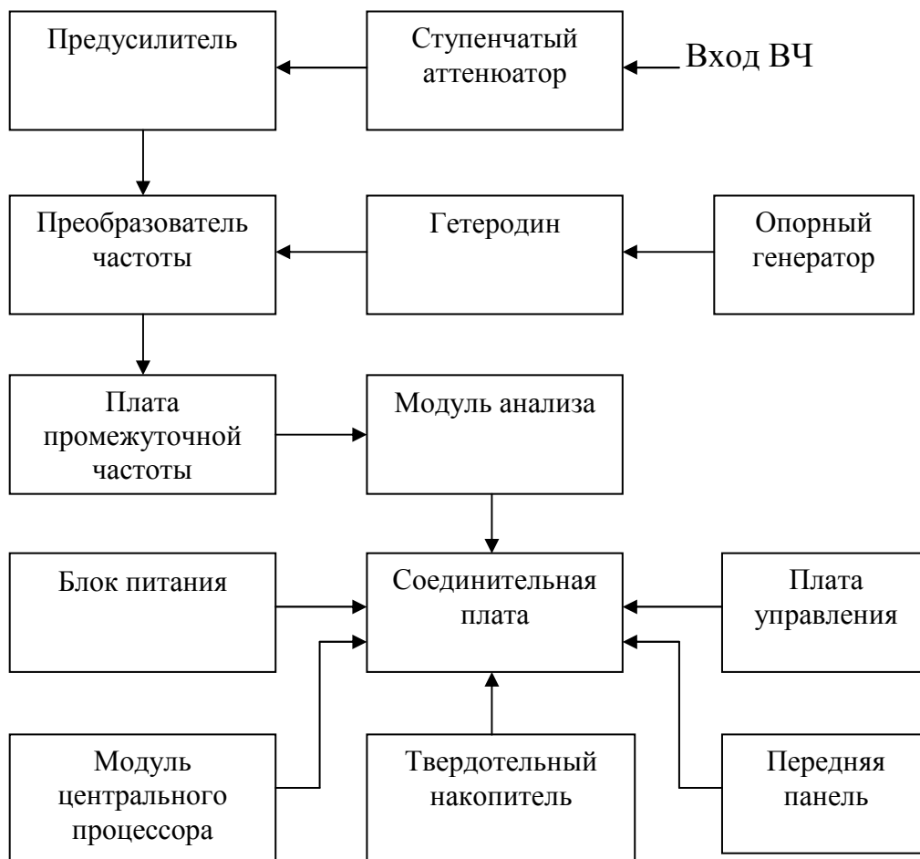
Рисунок 2. Структурная схема SPN9003A
