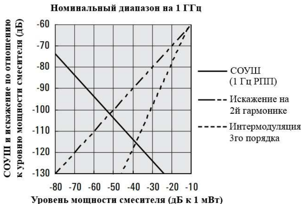
Рисунок1. Номинальный динамический диапазон, 9 кГц ... 3,6 ГГц
